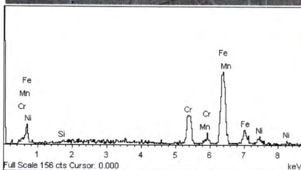
Εικόνα 66: Ενδεικτικές μικρογραφίες SEM και στοιχειακές αναλύσεις EDS Δείγματος "K5"
